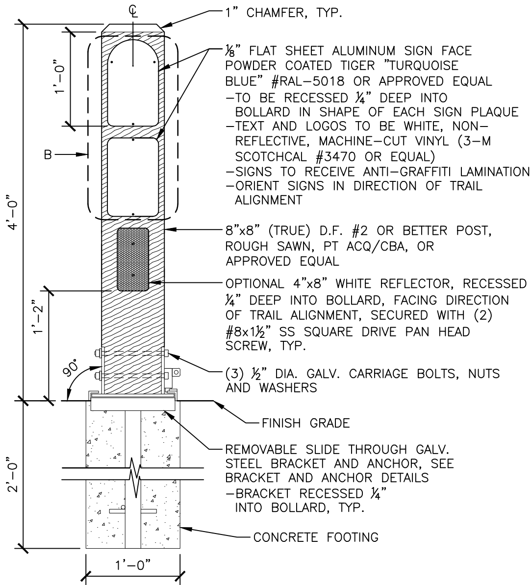
A-BOLLARD DETAIL
