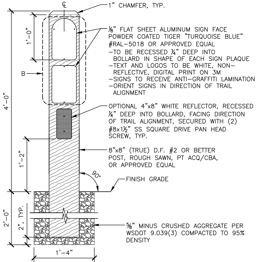
A-BOLLARD DETAIL
