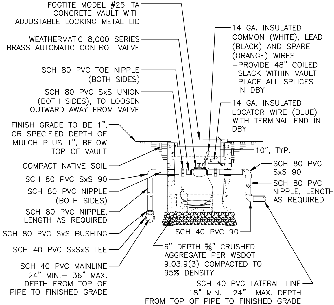
A-SECTION
